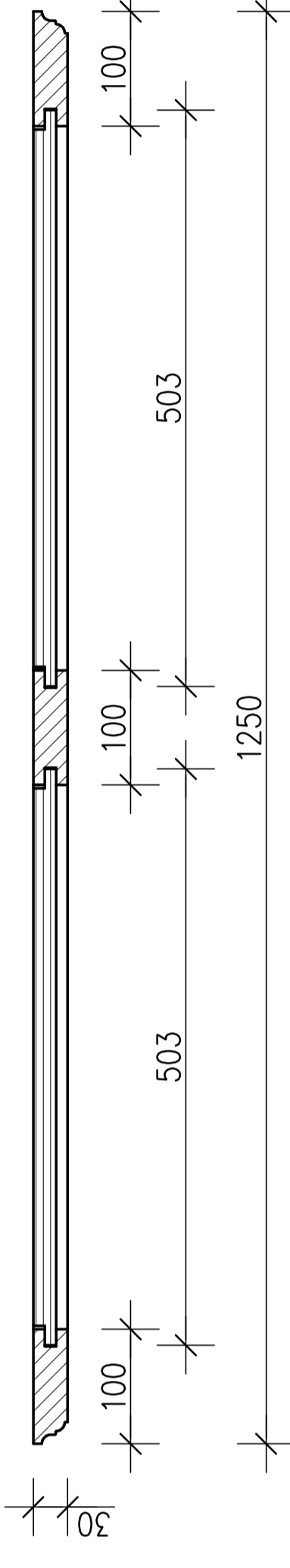
Schnitt Deckel A1-A2 M1:5
