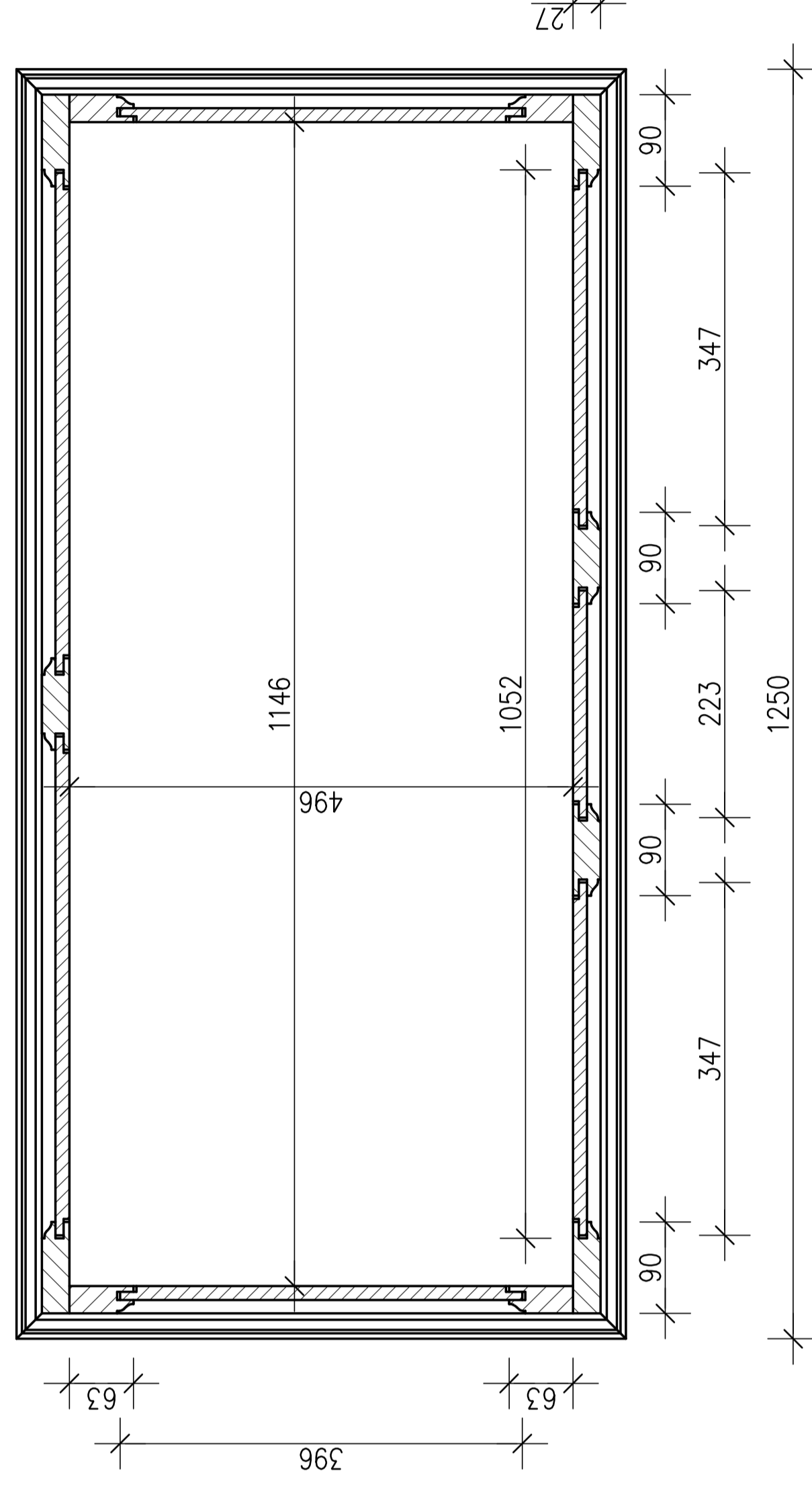
Schnitt G1-G3 M1:5
