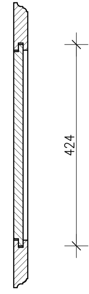
Schnitt Deckel S3-S4 M1:5
