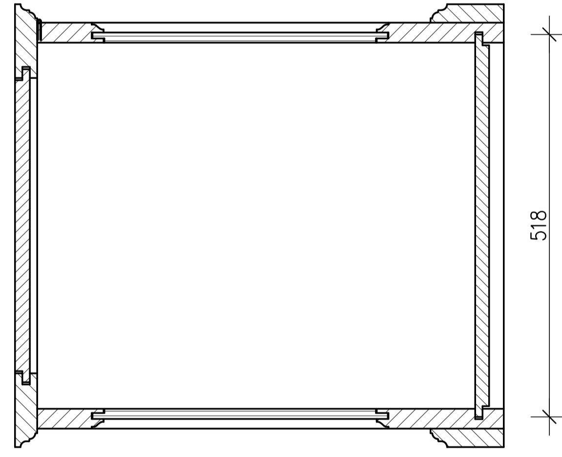
Schnitt S1-S2 M1:5
